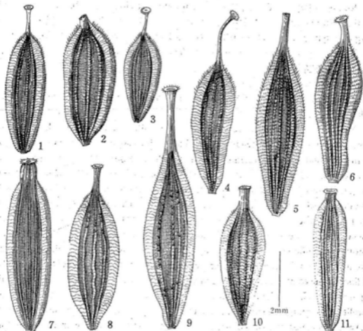
图1 毛瓣菊属与细莴苣属一些种的瘦果示意图 Achenes of some species of Chaetosaris and Stenosaris 1. 川甘毛瓣菊 Chaetosaris roborowskii ; 2. 蓝花毛瓣菊 Ch. cyanea ; 3. 菱裂毛瓣菊 Ch. rhombiformis ; 4. 栉齿毛瓣菊 Ch. pectiniformis ; 5. 光苞毛瓣菊 Ch. leirolepis ; 6. 大花毛瓣菊 Ch. grandiflora ; 7. 细莴苣 Stenosaris graciliflora ; 8. 粗毛毛瓣菊 Chaetosaris hispida ; 9. 戟裂毛瓣菊 Ch. taliensis ; 10. 滇藏毛瓣菊 Ch. hastata ; 11. 大理细莴苣 Stenosaris taliensis . (王金凤绘 drawn by Wang Jin-feng)
