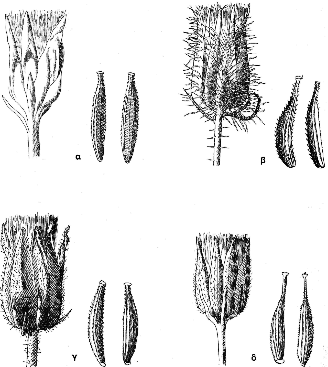
Είη. 3Α. Κεφάλια έν καρποφορία καί άχαύνια (περιφερειακά καί έπίδύσκια) τών: α, C. neglecta subsp. neglecta . β, C. neglecta subsp. corymbosa . γ, C. hellenica καί δ, C. cretica (Σχέδια Η. Lünser).
