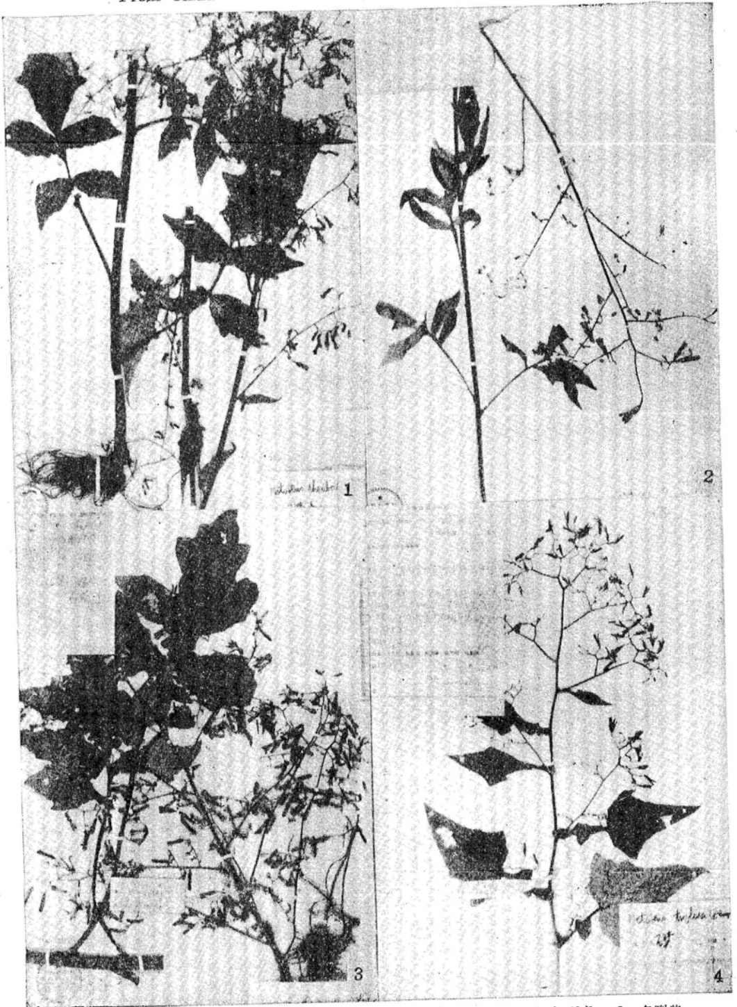
1. 菱叶紫菊 Notoseris rhombiformis Shih; 2. 南川紫菊 N. porpyrolepis Shih; 3. 多裂紫菊 N. henryi (Dunn) Shih; 4. 三花紫菊 N. triflora (Hemsl.) Shih.
