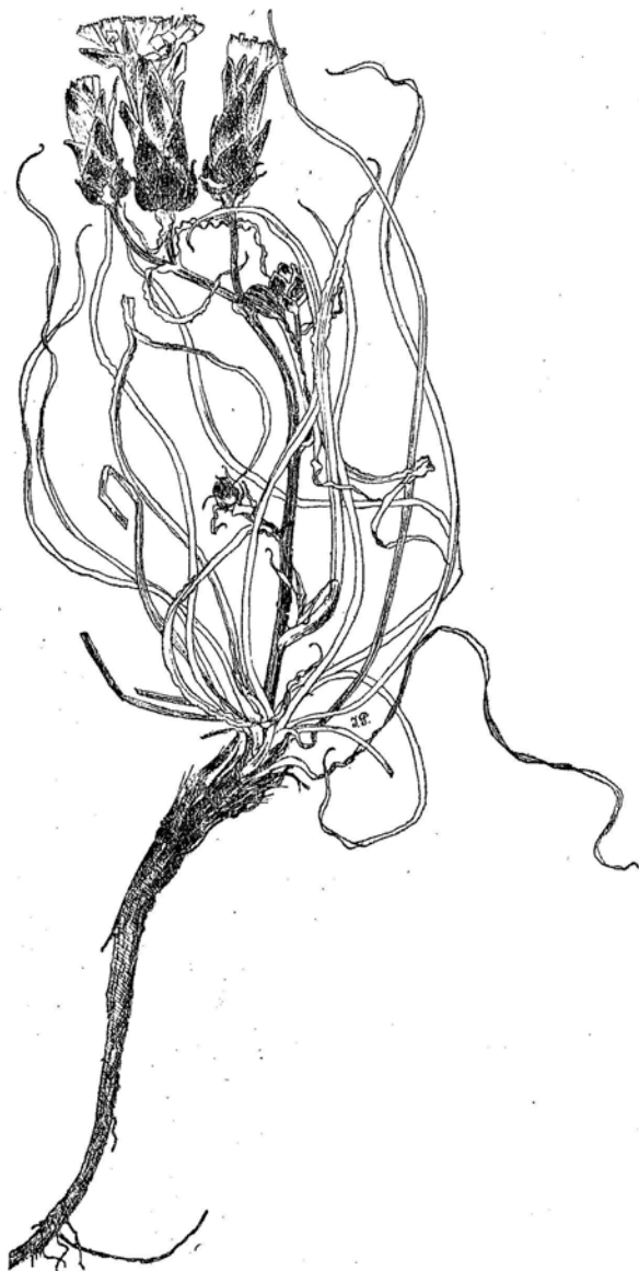
Fig. 1. Scorzonera baldschuanica Lipsch. sp. nova.
